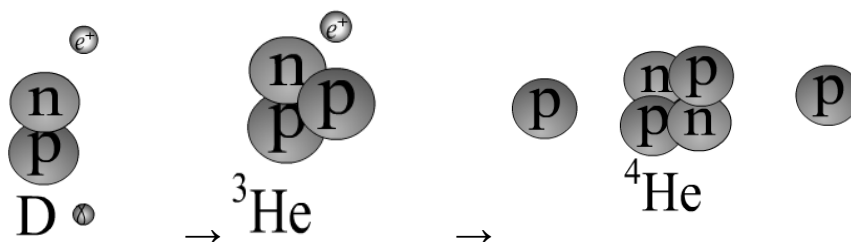
Рис.3. Синтез речовини
