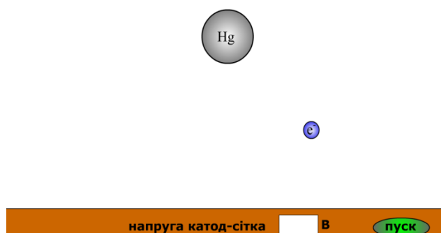
Рис.5. Бомбардування електронами атома ртуті
