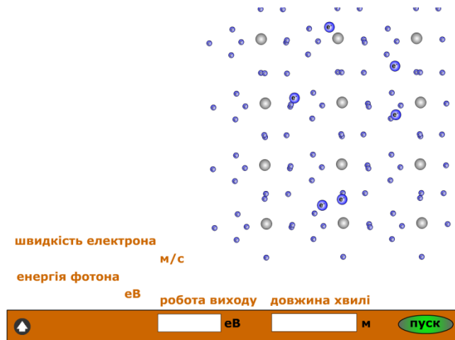
Рис. 4. Фотоефект
