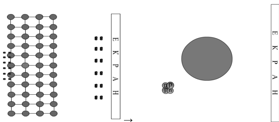
Рис.1. Бомбардування альфа частинками золотої пластинки
