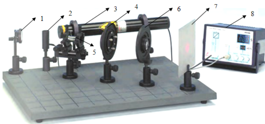
Рисунок 1 Установа для дослідження кілець Ньютона: 1 -лінза; 2 – магнітна стопа для оптичної лави; 3-лазер; 4- лінза; 5 -утримувач; 6-лінза; 7-екран; 8-джерело живлення
