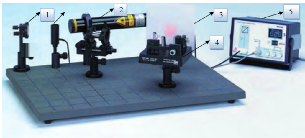
Рисунок 2 Інтерферометр Майкельсона на оптичній базовій платформі: 1- лінза; 2- інтерферометр Майкельсона; 3- екран; 4- магнітна стопа для оптичної базової платформи; 5 – джерело живлення
