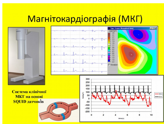
Рис. 1. Магнітокардіографія
